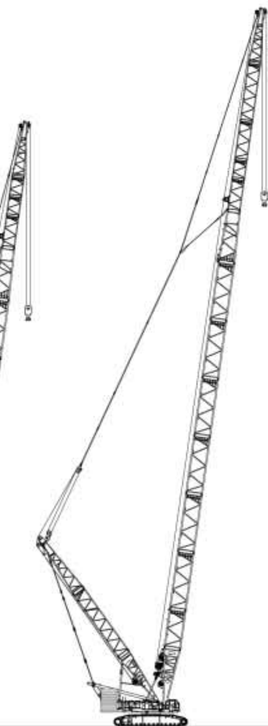
HL-ロング主ブーム
