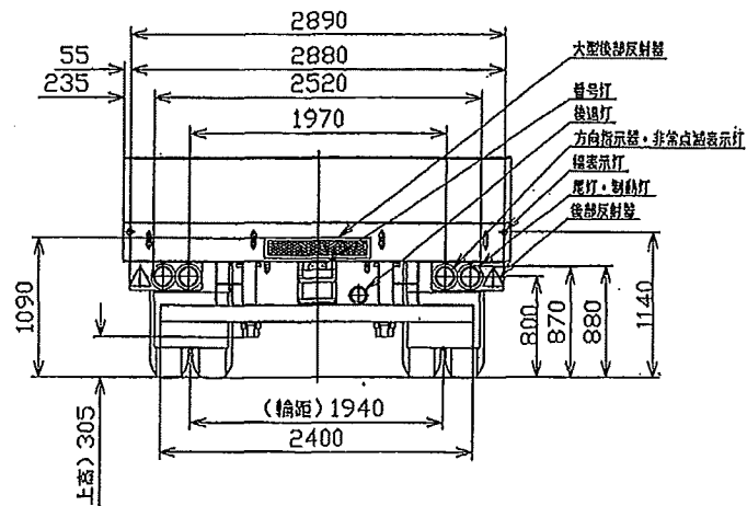
東急TL44J1C3S型セミトレーラ 外觀四面図
